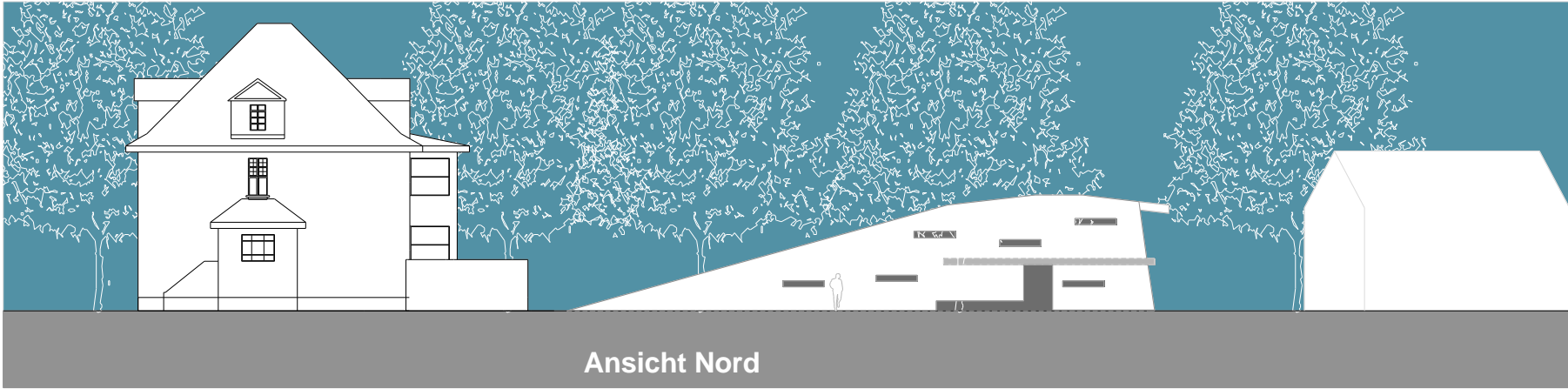
Schnitt A-A
